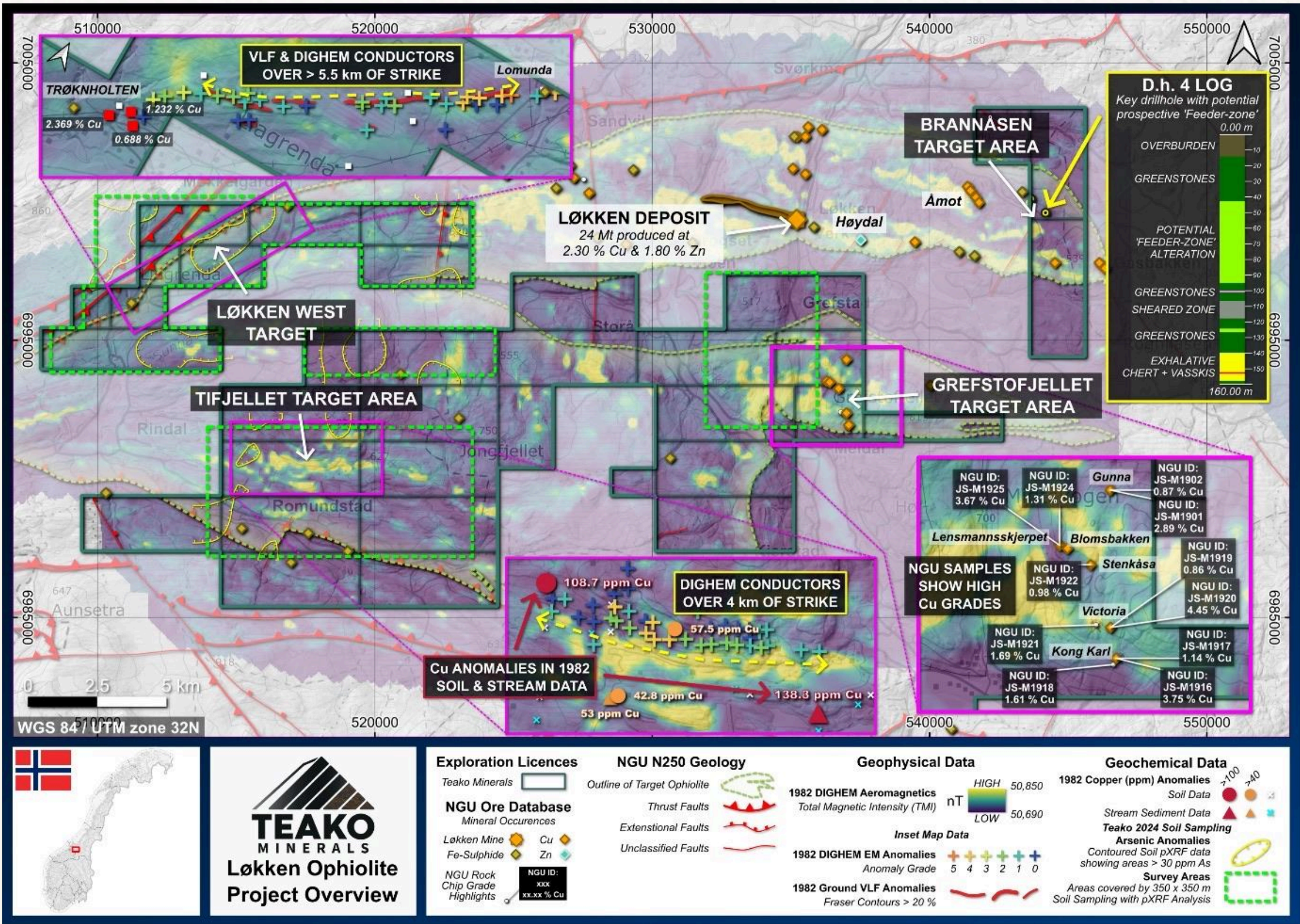
FIG. 18 · LØKKEN OPHIOLITE PROJECT OVERVIEW
