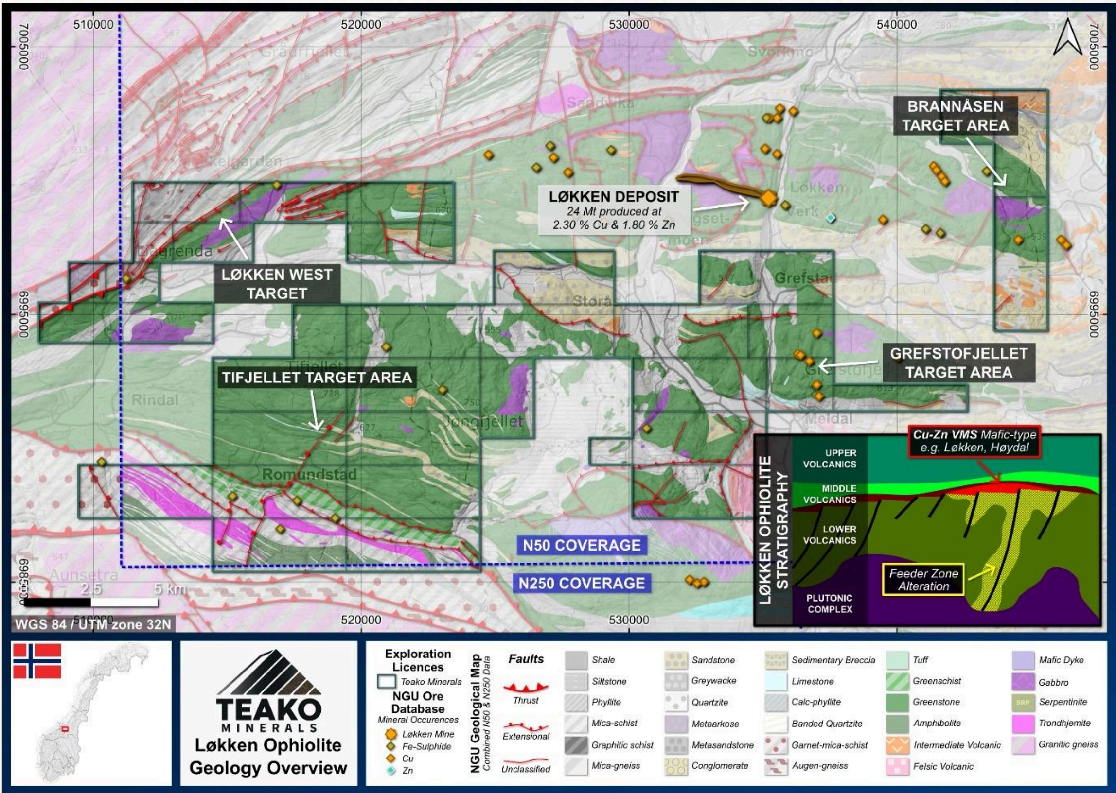
FIG. 19 · LØKKEN OPHIOLITE GEOLOGY OVERVIEW
