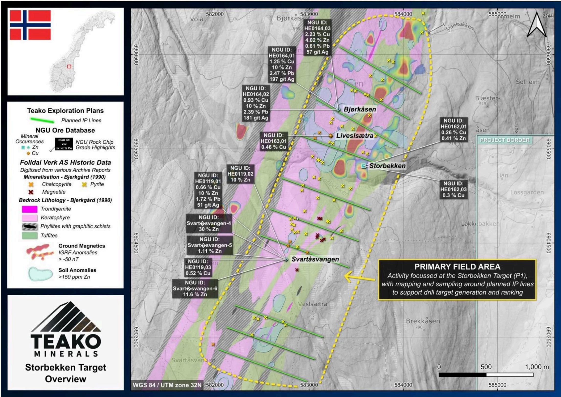
FIG. 12 • STORBEKKEN TARGET OVERVIEW
